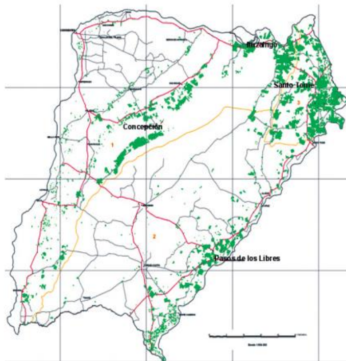
Figura 3. Distribución de las plantaciones forestales de la provincia de Corrientes; Fuente: DRF, 2009.
